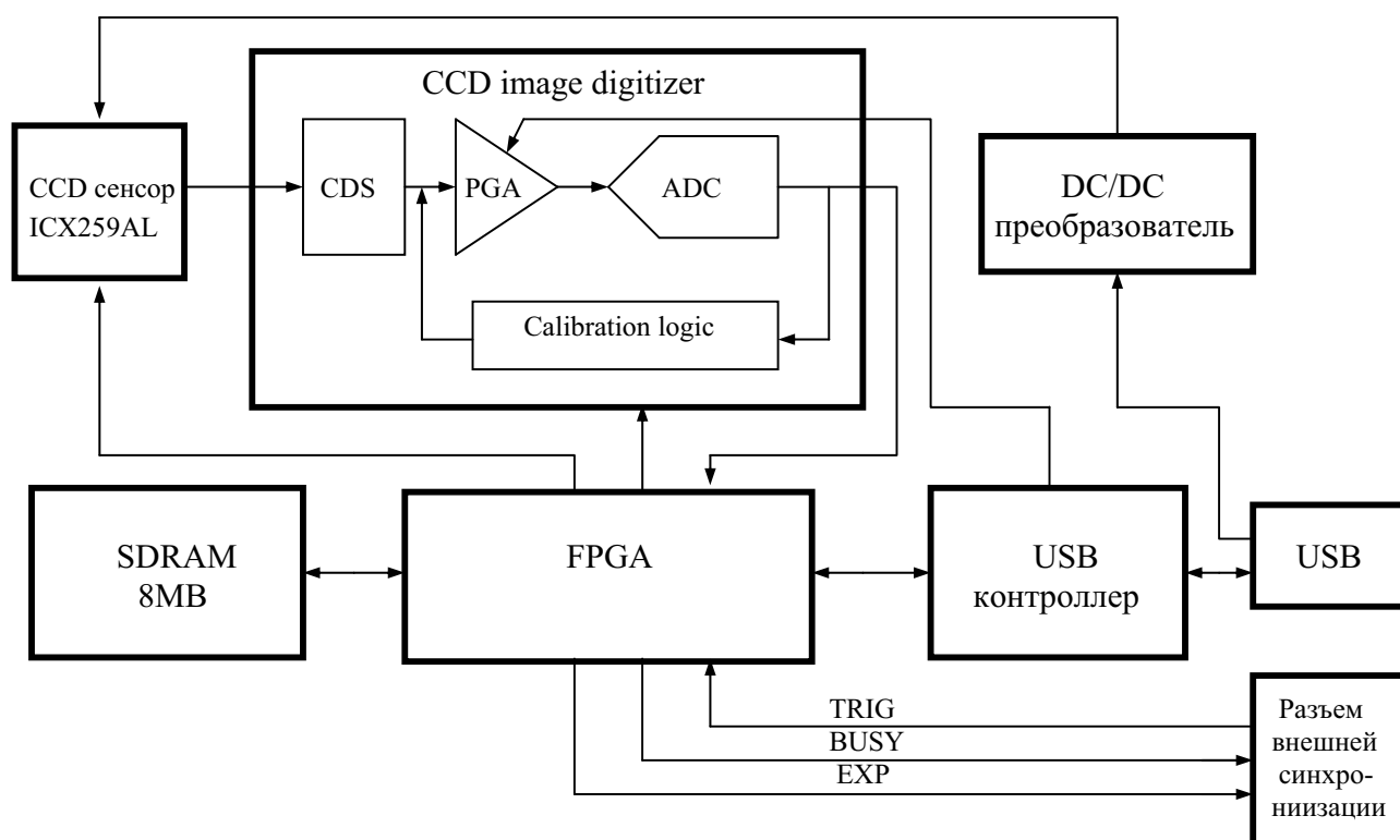
Рис. 1 Структурная схема камеры SDU-259
